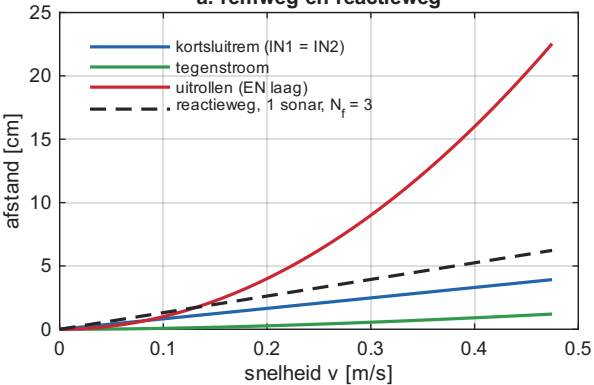
a. remweg en reactieweg
