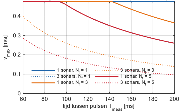
b. hoogste snelheid die F2.3 haalt (kortsluitrem)
